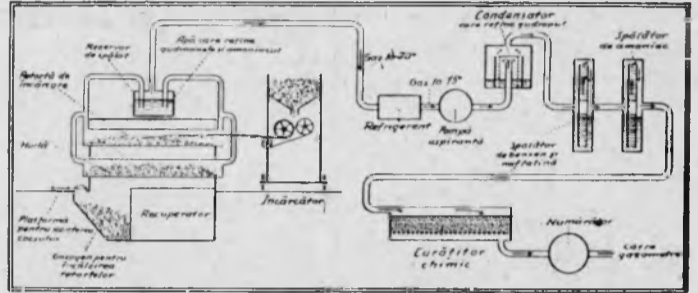
Schema distilării cărbunelui de pământ
