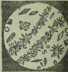
Hugysav kristályok
