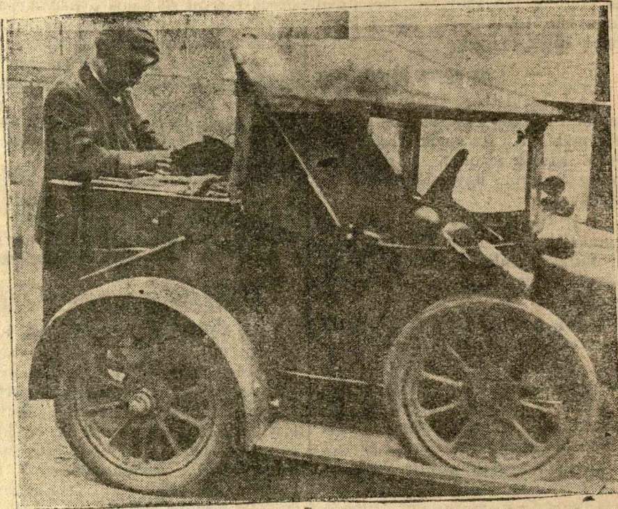
Valóban a technika haladásának kell mondani, hogy Franciaországban az uccai kőszörűsök is autózemre rendezkednek be. Képünk egy ilyen autóra felszerelt modern vándorló kőszörűsműhelyt mutat be.
