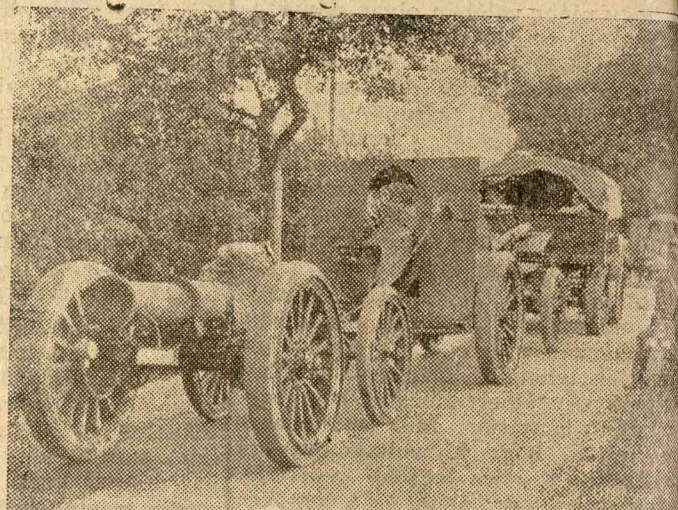
TÜZÉRSÉGI NEHÉZ ÁGYUK szállítása a francia hadsereg számára
