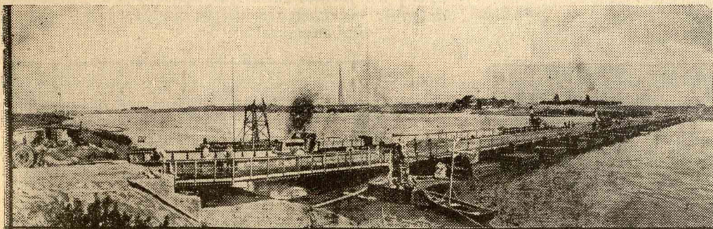
A VISZTULA UJ HIDJA DANZIG MELLETT. Danzig szabadállam hatalmas hidat épített a Visztula folyón át. Képünk a hidépítési munkálatok befejezését ábrázolja.
