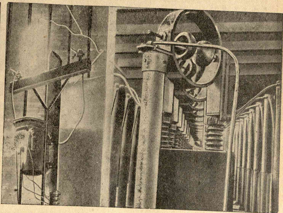
KISÉRLETEK 3 MILLIÓ VOLTAL. Az egyik amerikai kísérleti telepen most érdekes kísérletek folynak oly irányban, hogy 3 millió voltos áramot szikra alakjában vezessenek át transzformátorokba és áramgyűjtőtelepekbe.
