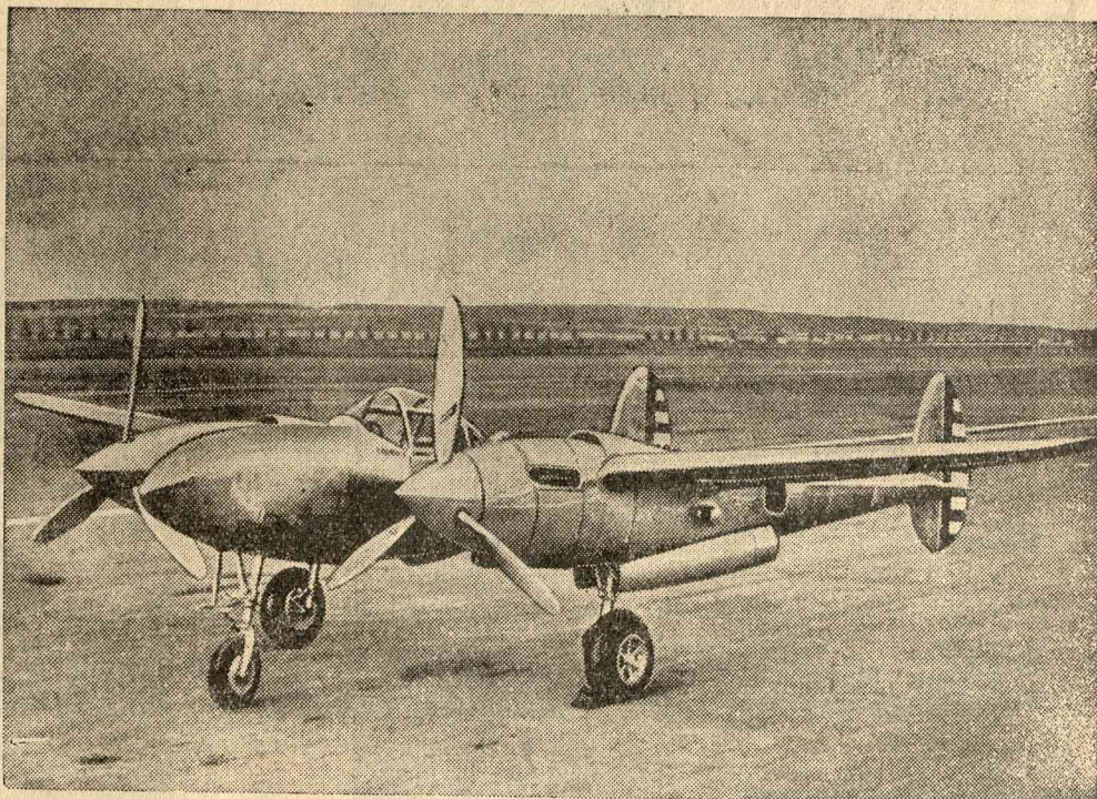
UJTIPUSU AMERIKAI VADÁSZREPÜLŐGÉP. Ez a repülőgép óránként 570 kilométeres sebességet tud kifejteni.
