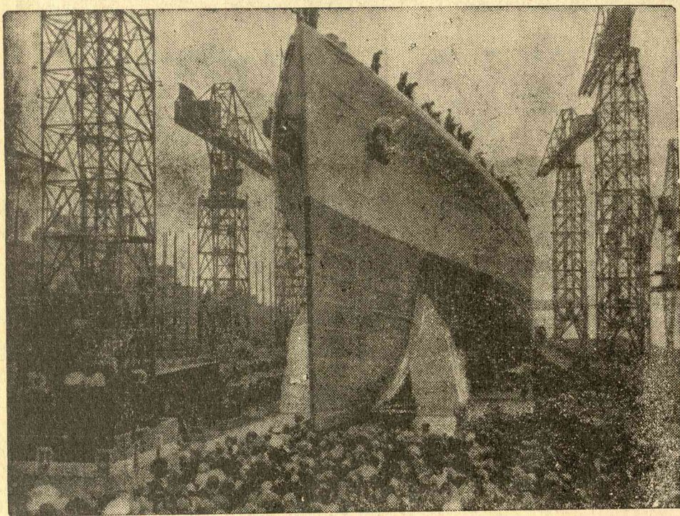
ANGLIA LEGNAGYOBB ÉS LEGUJABB HADIHAJÓJA. Negyven-ezer néző előtt bocsátották vízre Anglia legnagyobb és legmodernebb csatahajóját, a 35.000 tonnás Prince of Walest.
