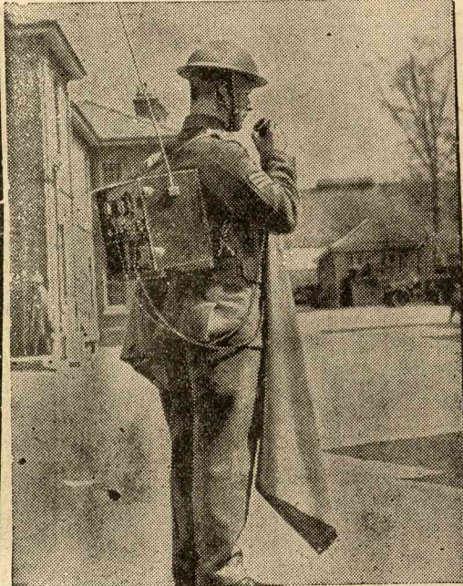
HORDOZHATÓ SZIKRATÁVIRÓ. Az angol hadseregben most mutatták be a hordozható szikratávirót, amely állítólag kitűnően bevált.
