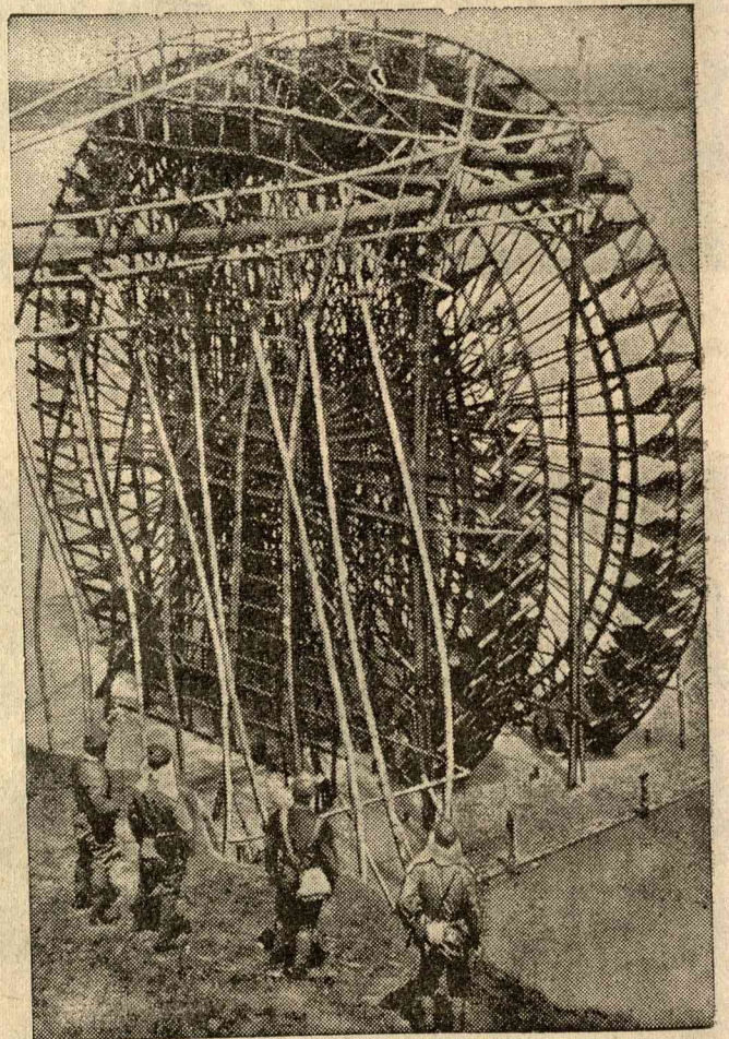
ÓRIÁS VIZKERÉK HAININ SZIGE- TÉN. Hainan szigetén óriási kerekeken emelik a magasba felállított csator- nába a vizet, amely a földek öntözé- sére szolgál.
