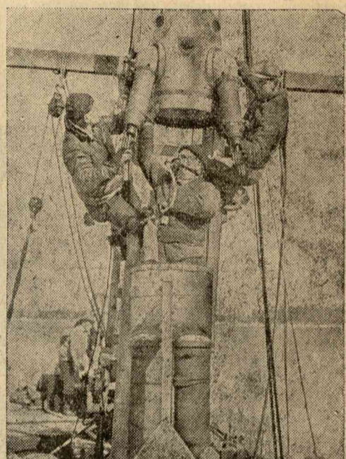
BUVÁRÖLTÖZÉK 800 MÉTER MÉLYSÉG SZÁMÁRA. Egy Baumann nevezetű amerikai óceánmélység-kutató a képünkön látható buváröltözéket készítette el, amely alkalmassá teszi 800 méteres mélységbe való leszállásra.
