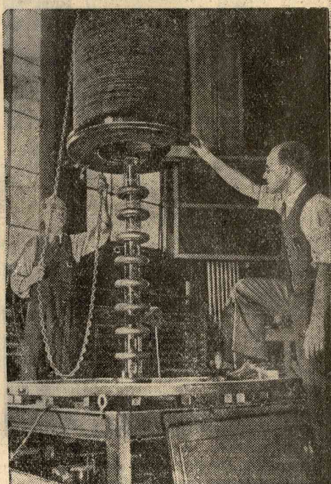
A VILÁG LEGNAGYOBB RÖNTGEN-CSÖVE. Schenectady-ben építik meg a világ legnagyobb Röntgen-csővét, amely egymillió voltos lesz.
