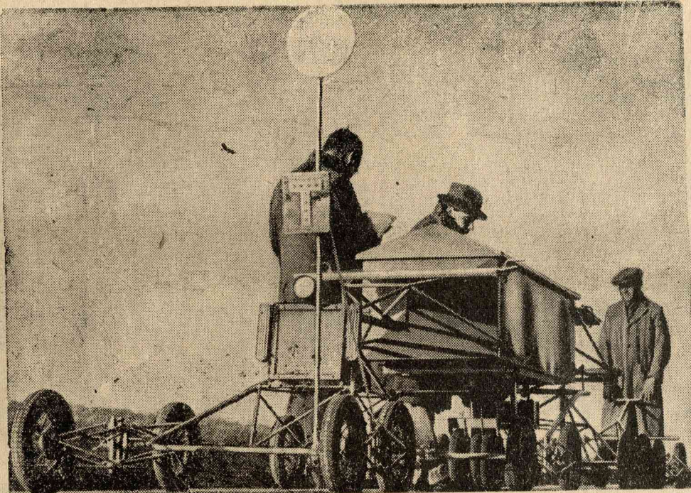
UTEGYENETLENSÉGI SZABÁLYOZÓ. Az utak egyenetlenségét a képünkön látható 16 kerekes rendkívül érzékeny szerkezettel mérik Angliában.
