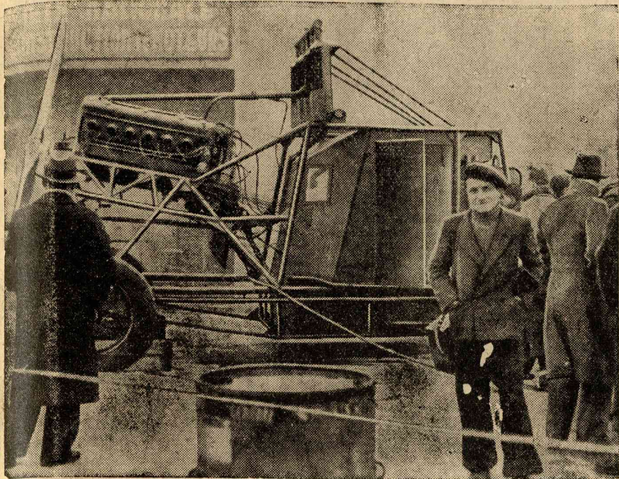
REPÜLŐGÉPMOTORVIZSGÁLÓ INTÉZETET ÁLLITOTTAK FEL A MONT BLANCON. A francia repülésügyi miniszter rendeletére Mont Lachat-on 2100 méter magasságban motorvizsgáló intézetet állítottak fel, amelynek célja a motorok nagy magasságban való működésének megfigyelése.
