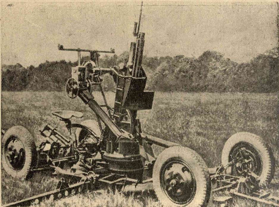
AMERIKA LEGUJABB LÉGELHÁRÍTÓ ÁGYUJA.
