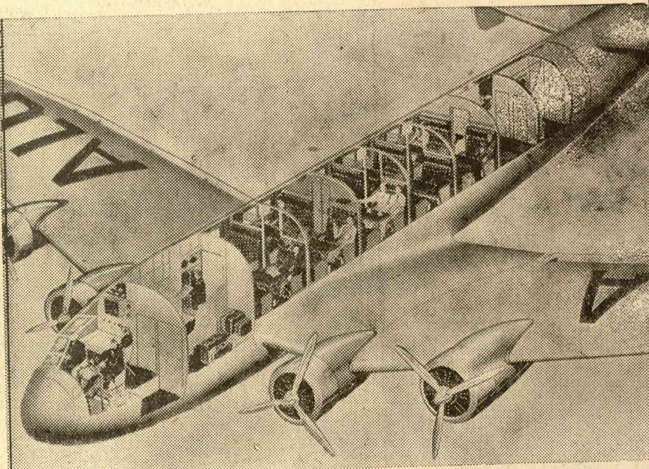
BEMUTATKOZOTT A LEGUJABB LUFTHANSA-GÉP. A Berlin-Tempelhof-i repülőtéren mutatkozott be a legujabb típusú I. 90. jelzésű repülőgép, amely 40 utast visz magával és 400 kilométeres óránkénti sebességgel halad.
