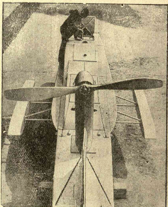
ÚJSZERŰ VIZIJÁRMŰ. René Morin, francia mérnök újszerű vizijárművet készített. Ezt a gépet egy propeller hajtja előre és 90 kilométeres óránkénti sebességet tud elérni. Rendkívüli előnye, hogy a hajótest nem mélyjárata és így a víz ellenállását könnyen le tudja küzdeni.
