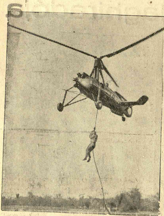
Légipropeller az egészségügy szolgálatban. Franciaországban próbálták ki először az u. n. autógiró egészségügyi szolgálatba való állítását.
