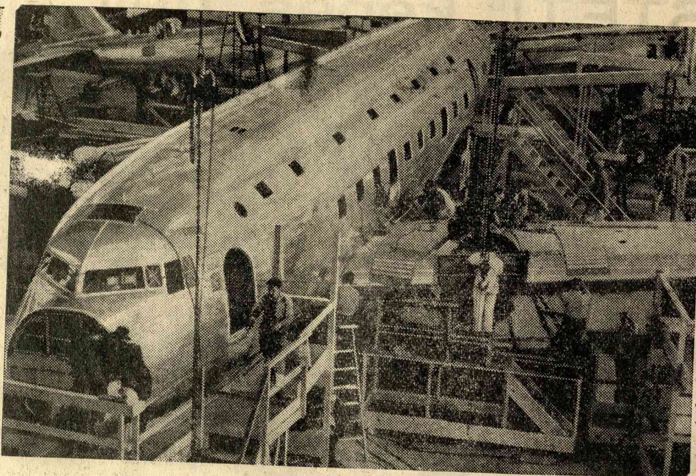
Óriásrepülőgép építés közben. Santa Monica-ban, Kaliforniában, készül ez az óriási, 42 utas szállítására alkalmas repülőgép, melyet 5600 lóerős motorok fognak hajtani
