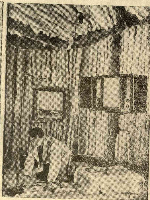
Hangos beszélő vattázott falak között. A hangos beszélőket, hogy tökéletesen kipróbálhassák, vattázott-falu szobában állítják fel.
