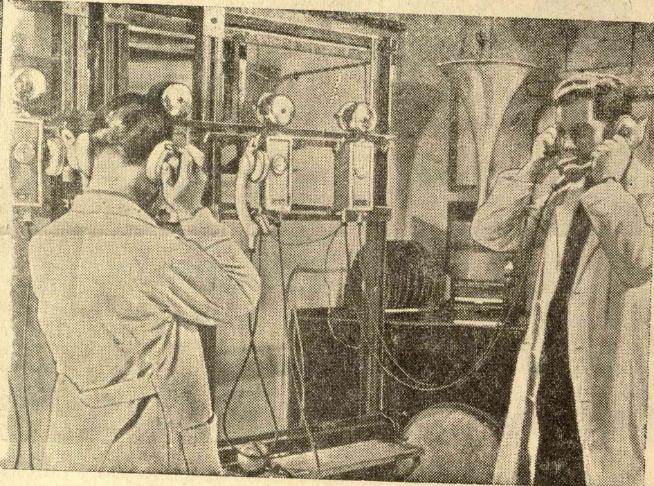
Telefonálás pokoli lármában. A berlini Siemens-Haske műveknél kísérletek folynak az irányban, hogy oly távbeszélő-készülékeket készítsenek, mely minden pokoli lármában is lehetővé tegye a távbeszélést.
