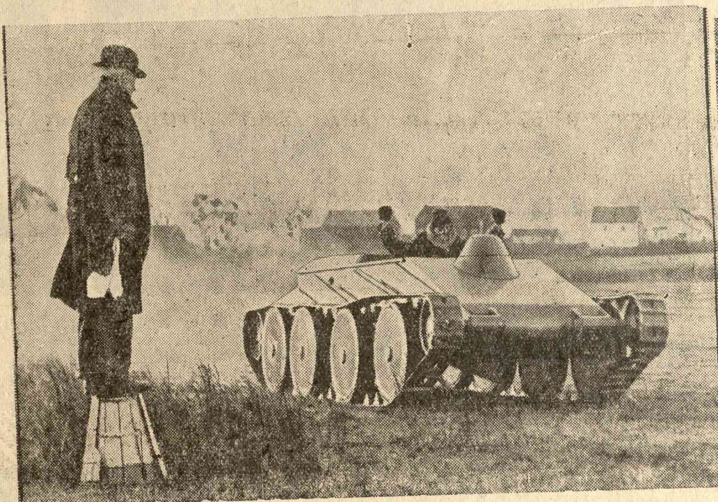
Új amerikai tanktipus. A hetvenéves amerikai mérnök, Walter Christie a ké- pünkön látható új tanktipust készítette el. A gép 140 mázsa súlyú és egy 430 lóerős motor hajtja óránként 90 kilométeres sebességgel.
