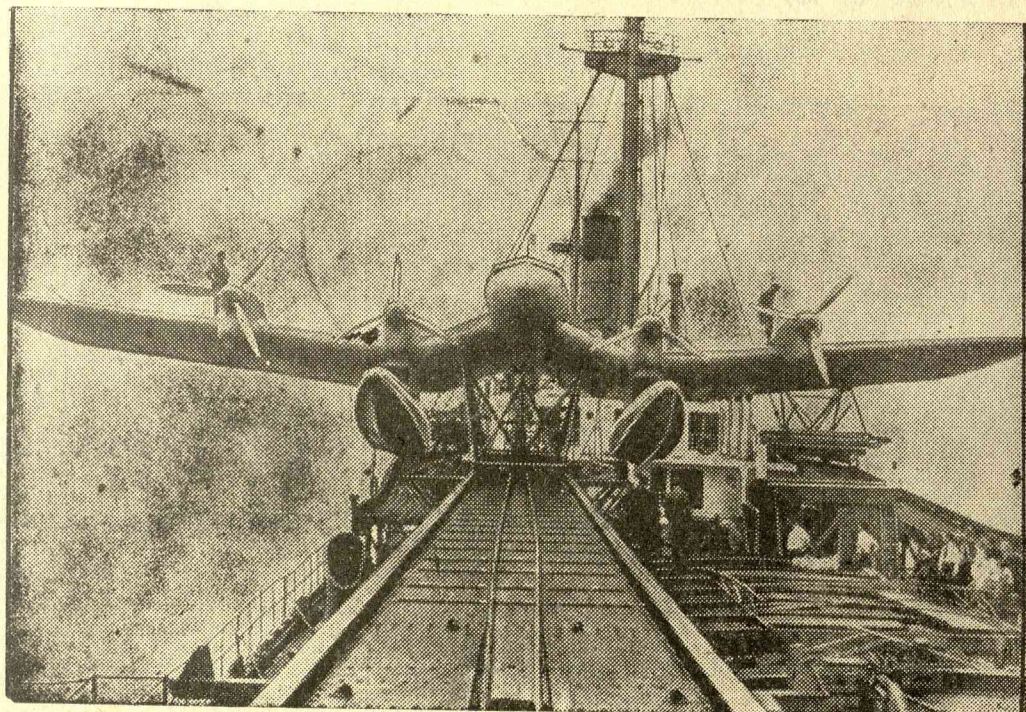
A Lufthansa kísérleti gépe a Nordmeer, mely már több ízben repülte át megállás nélkül az óceánt.
