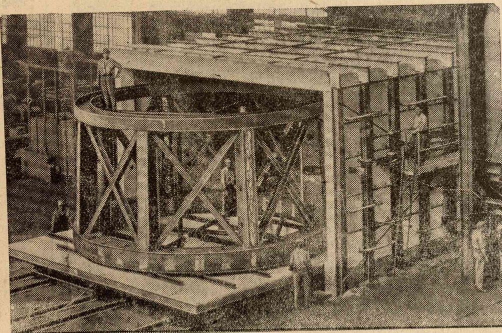
A világ legnagyobb teleszkopja. A kaliforniai Palomar csillagvizsgálóban álli- tották fel a világ legnagyobb csillagászati látcsövét. Átmérője 22 láb, vastag- sága 12 láb. A hatalmas méretű látcső lencséjének foglalatát mutatjuk be.
