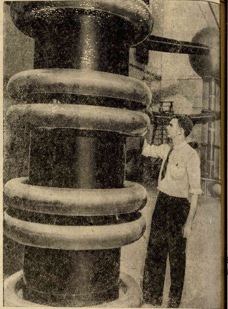
Egy millió volt. Dr. Crane, a Michigan egyetem fizikusa egy olyan készüléket konstruált, amelyet egy millió volt töltethetnek meg. Képünk a nagy elektromos rezervoár ábrázolja.
