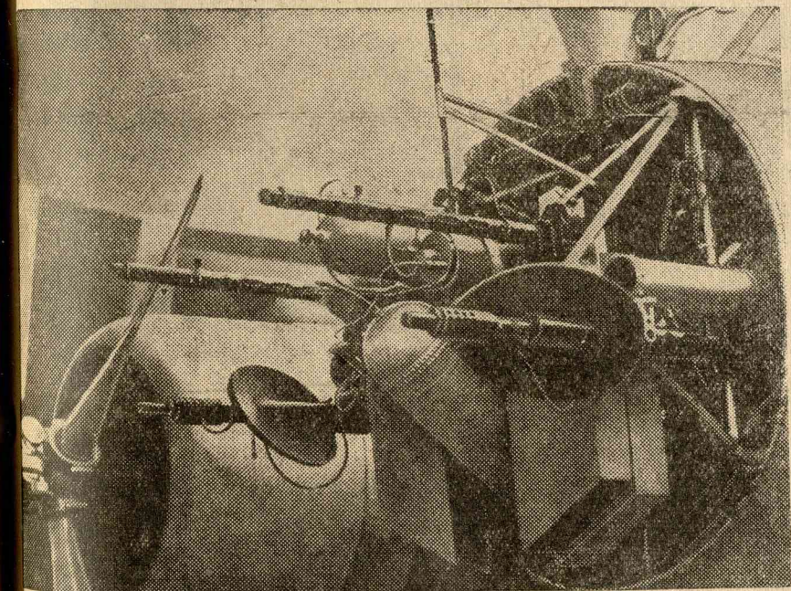
Igy fest egy Focke-motor. A párisi kiállításon látható a fenti Focke, mely két 23 milliméteres gyorstűzelő ágyúval és két 7.3 milliméteres gépfegyverrel van felszerelve.
