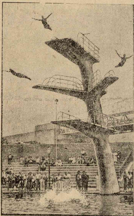
Fa-alaku ugróhid. A newyorki Astoria-uszodában a képünkön ábrázolt fa-alaku ugróhidat készítették.
