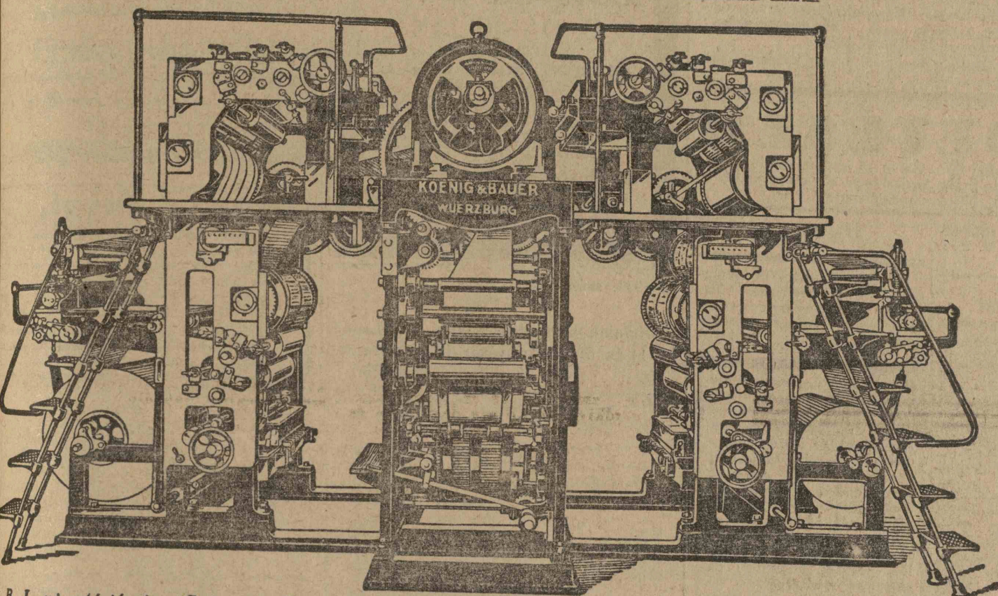
A. B. L. új rotációs gépe. Gyártotta: Koenig et Bauer Schnellpressenfabrik A. G. Würzburg. Vezérképviselet Románia részére: Henry et Emanuel Fränkel, Bukarest I.
