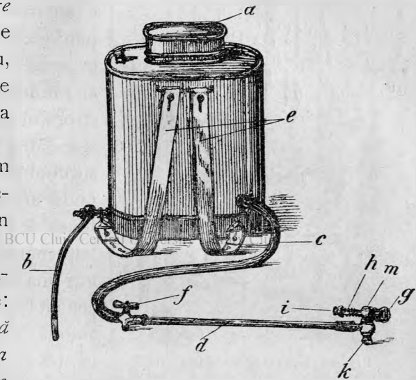
Fig. 43. Pumpă de stropit.
