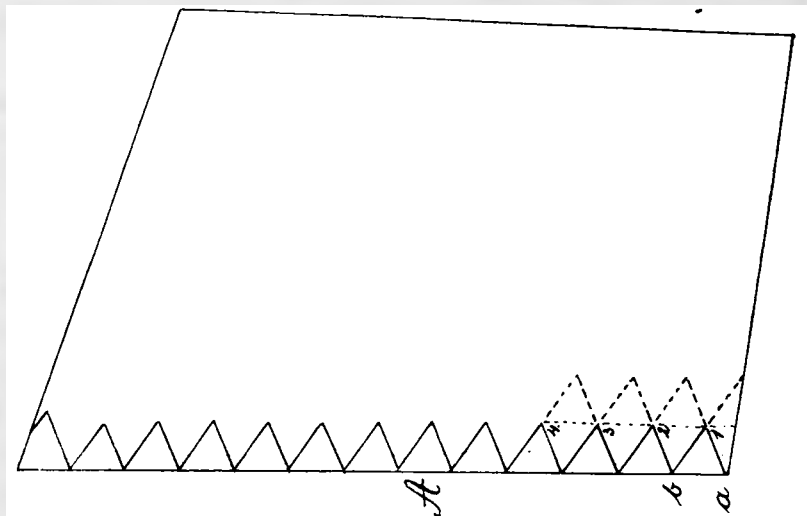
Fig. 3. Fixarea sau insemnarea depărtării rândurilor și a vițelor pe un teren cu figură neregulată, cu ajutorul triunghiului.
