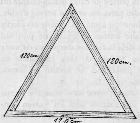
Fig. 4. Triunghi pentru fixarea depărtării rândurilor și a vițelor, buciunilor, buturelor intru sine.
