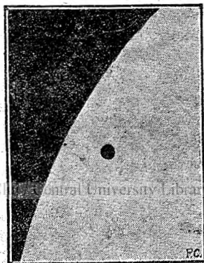
Fig. 4.— Trecerea lui Mercur peste discul soarelui la 8 Mai 1924.
