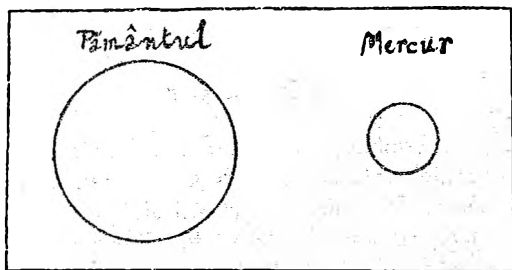
Fig. 2. — Mărimea pământului față de Mercur.
