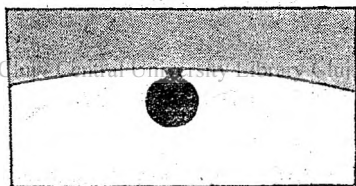
Fig. 8. — Trecerea lui Venus peste discul solar: Picătura neagră.
