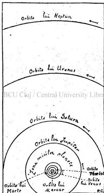
Fig. 1. — Sistemul planetar.
