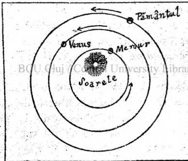
Fig. 3. — Orbitele lui Mercur și Venus sunt înăuntrul orbitei pământului.
