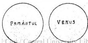
Fig. 7. — Pământul și Venus.
