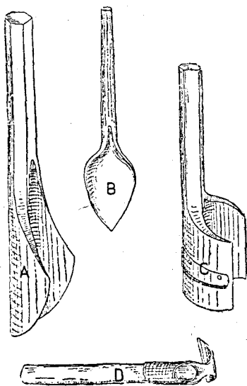
12. kép. Pinus-félék csapolásához szükséges szerszámok. A Kúpos véső a gyűjtőgödörhez, B vaskanal a balzsam kiszedéséhez, C íves véső a pléhlap berakásához, D kaparó a gyanta gyűjtéséhez. (Az Erdészeti Kísérletek 1917. évi 1—2. füzetéből.)
