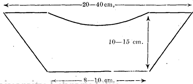
6. kép. Pléből készült kötény az amerikai gyantacsapoláshoz. (Az Erdészeti Kísérletek 1917. évi 1-2. füzetéből.)
