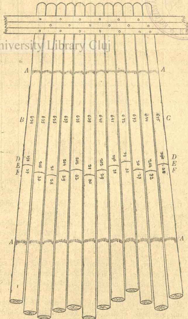
A. Festéksáv. — B. Legkisebb szám. — C. Legnagyobb szám. — D. Hosszúsági méret. — E. Középvonal. — F. Vastagsági méret
