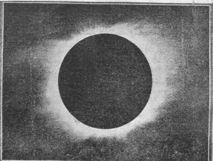
Eclipsa totală de Soare, care s'a produs la 28 Maiu, 1900, și fotografiată de Yerkes. Razele albe sunt coroana Soarelui
