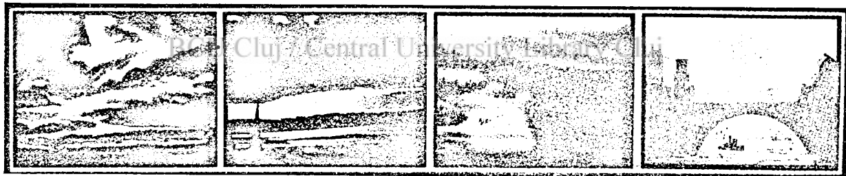
Nourii în forma aceasta au o aparență amenințătoare, dar de fapt sunt prevestitorii vremii bune și frumoase.
