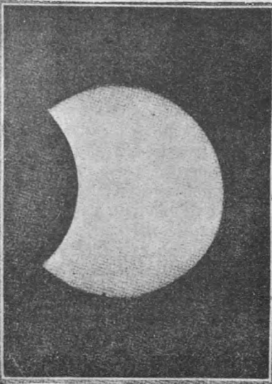
O altă privire a eclipsei, care e și mai mică ca cea premergătoare.
