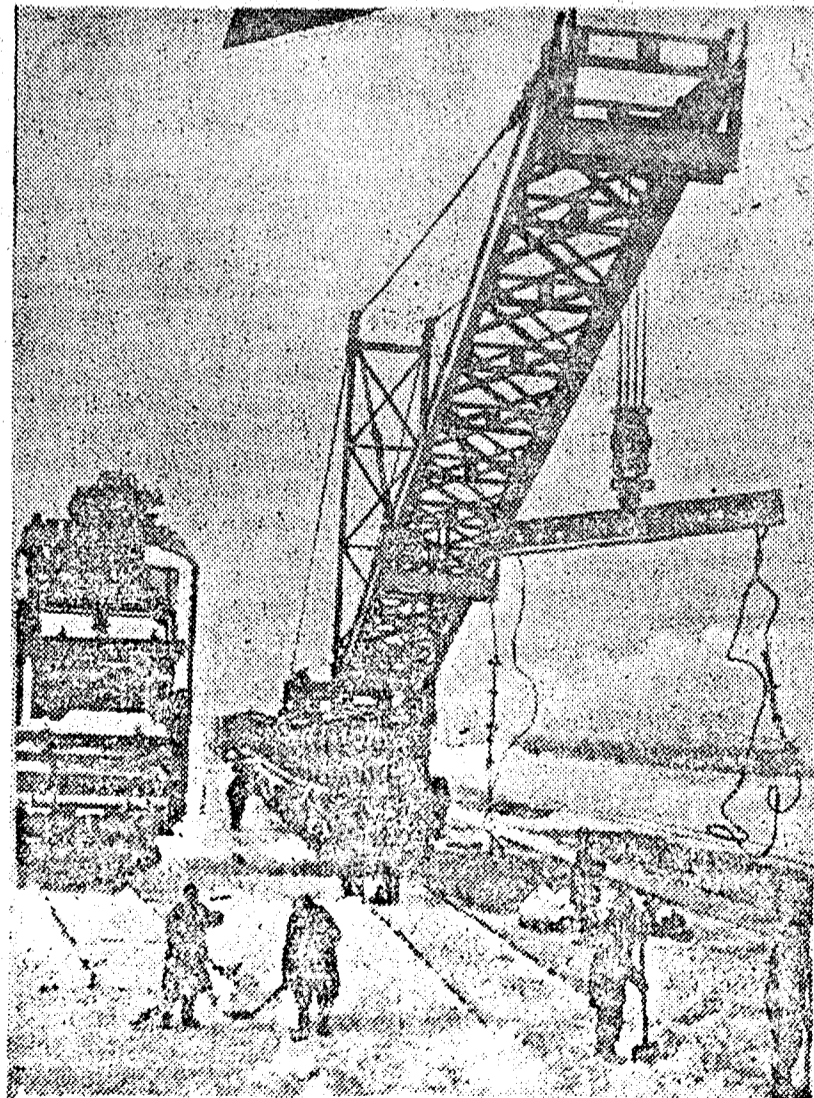
A kujbisevi víztorony építő-telepein vasuti hálózatot létesítenek. Ez a munka nagyteljesítményű gépekkel történik. A fenti képen egy vasut-építő gép készen áll az összerakott híd, a másik pedig vágányokat rak le.
