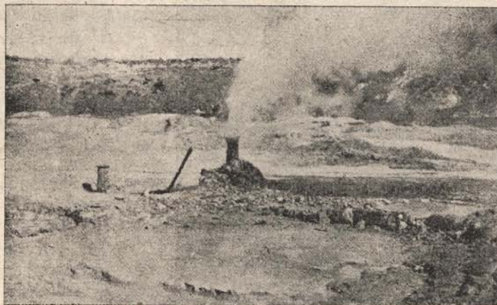
Vulcanul „La Solfatara“ din Pozzuoli, în Italia. Aparatul care se vede în ilustrația noastră servește pentru estragerea forței motrice din adâncul pământului. La dreapta coșului, ce fumegă, se află un puț, cu conținut ferbinte și care spumegă.
