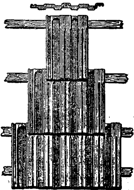
Țigle duble de siguranță tescuite de-ale lui Bohn, patentate cu Nr. 253. — Depărtarea lețelor 34 cm.
