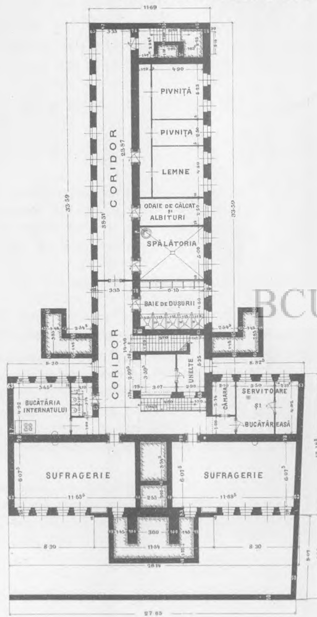
Subsolul
