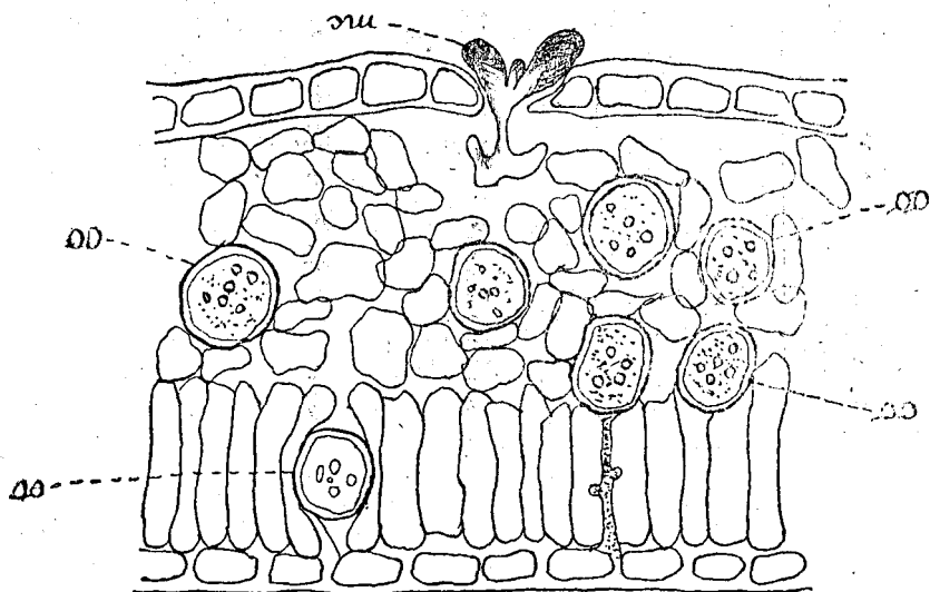
3. ábra. Egy szőlőlevél átmetszete, melyben 00-nál spórák képződnek.
