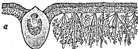
1. ábra. A szőlőlevél peronoszporájával.
