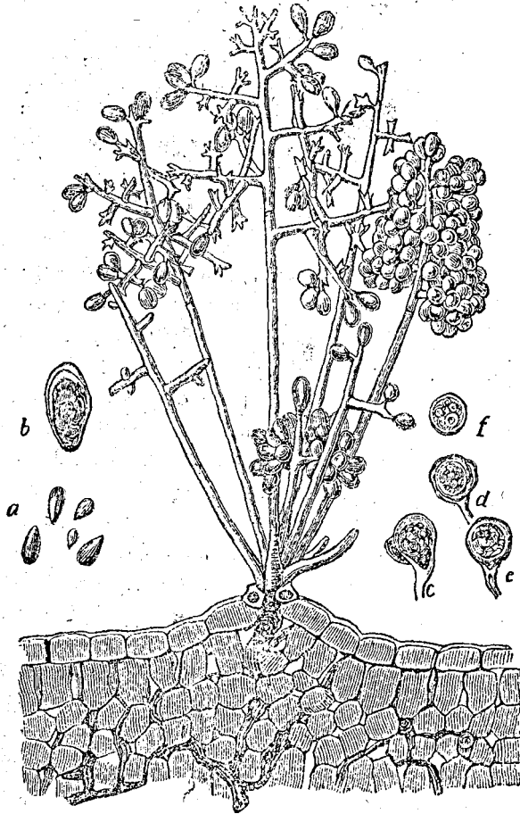
2. ábra. A csirasejtek vagy konidiumok keletkezése.
