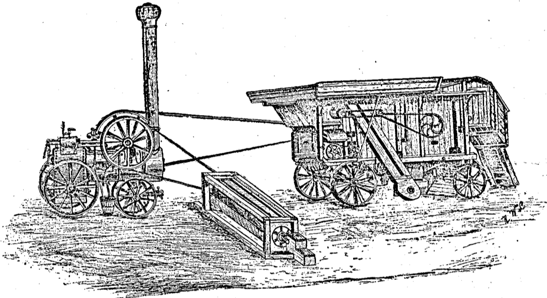
A heremag cséplése a Gerendy-féle eljárás szerint.
