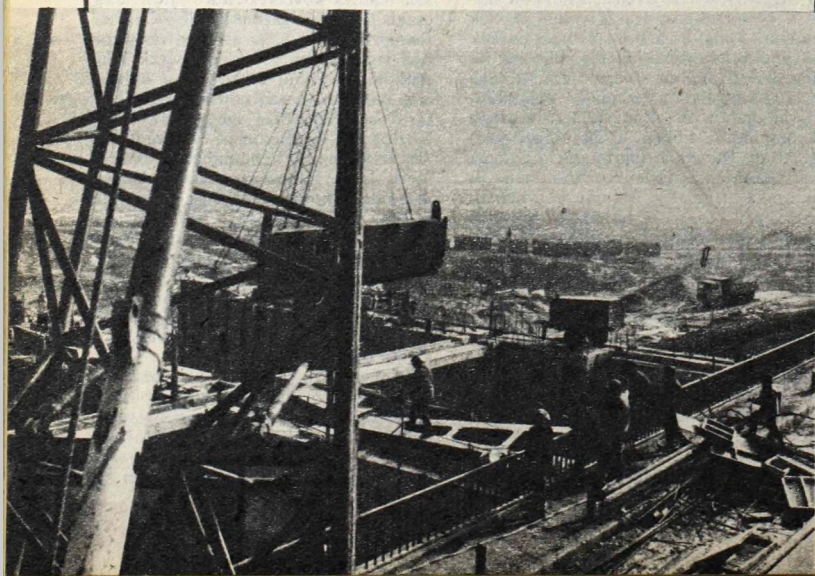
Az ötéves terv egyik nagy beruházása: az Arges folyó szabályozása
