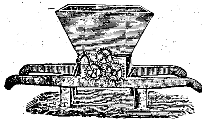
Fig. III. Strivitoare de struguri cu învîrtitor de mână, cu 50 cor. bucata.
