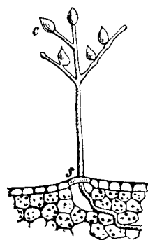
Fig. 4. Perenospora eșită din coaje, ca să rodească, c conidii.
