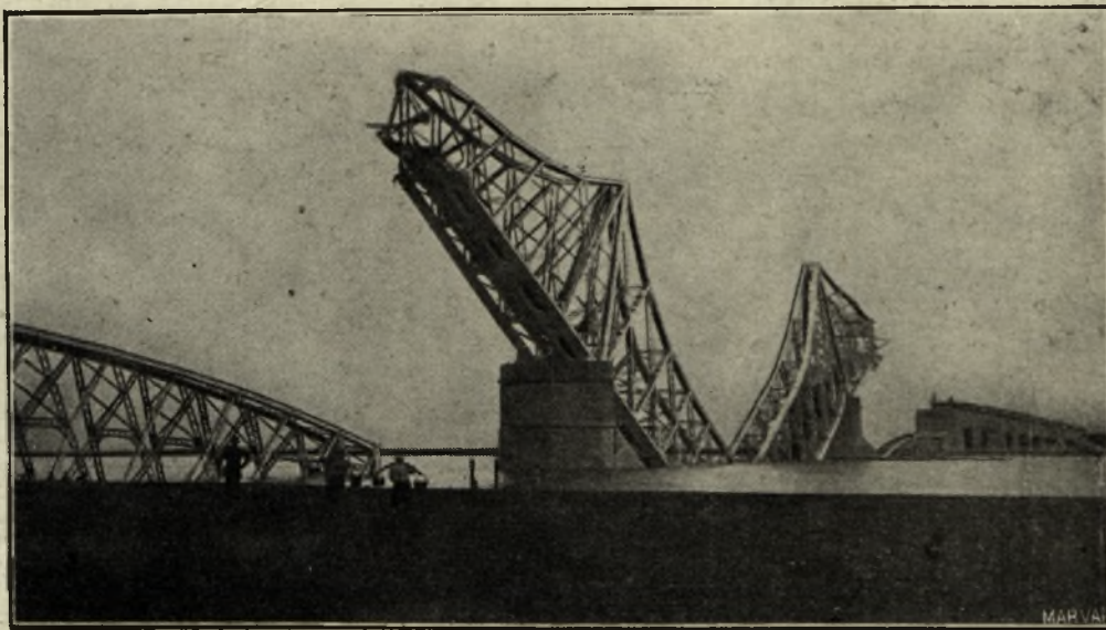
Podul de peste Dunăre (brațul Borcea) distrus în toamna anului 1916.
