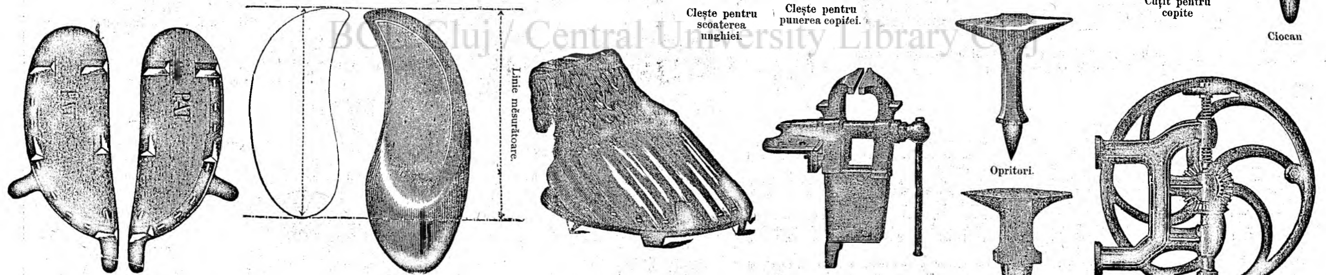
Fier de pus la unghii normal pentru vară și iarnă. Fierurile de iarnă au dinți și hacuri ascuțite, cele de vară tocite. La ori-ce potcovire de boi se ia măsura numai de pe partea din față a unghiei, și anume după-cum arată chipul de mai sus. Unghiile dinderept nu trebuie se să măsore. Fiind acestea peste tot ceva mai plane și virfuite; fierurile pentru ele se capătă după măsurătoarea copitelor din față.
