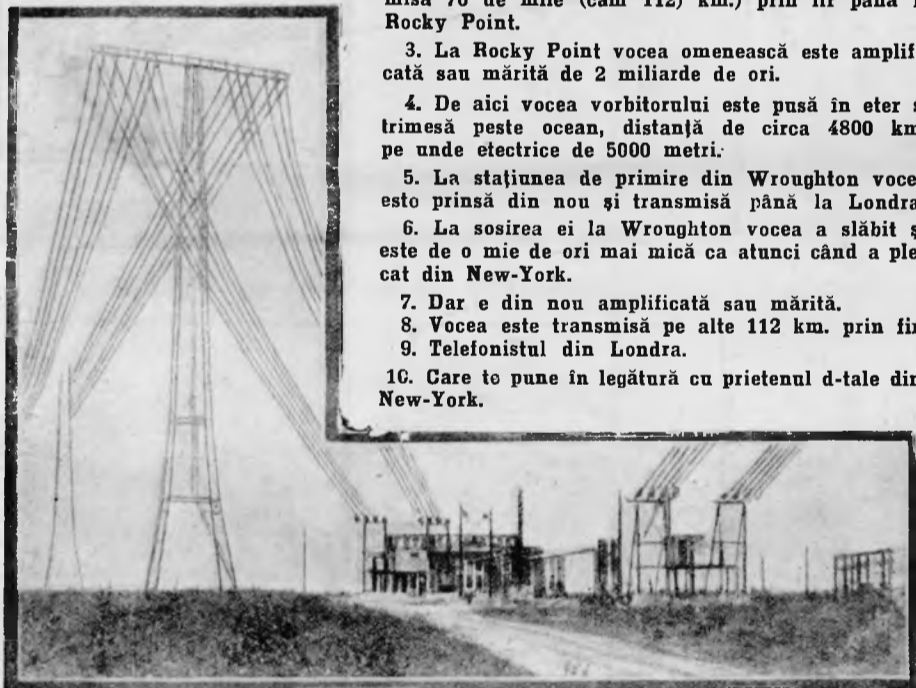
Stațiunea dela Rocky Point, Long Island (New-York) pentru primirea și transmiterea peste ocean a vorbirilor telefonice.
