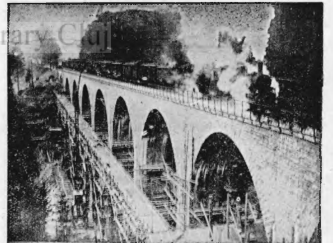
Cel mai mare pod de piatră din Europa. Acest pod are o lungime de 224 metri cu 9 arcade și se găsește în Munții Pădurea Neagră. Înălțarea lui a durat un an și jumătate și la 14 Decembrie a fost inaugurat. În timpul deceniului construcției de fier, podurile de piatră sunt tot mai rare
