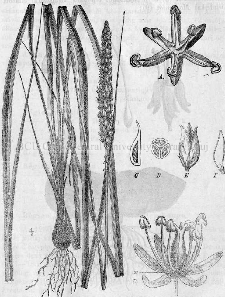
8. Schoenocaulon officinale (SCHLECHTENDAL) A GRAY. Habitus kicsiny. A ♂ vir., B ♀ vir. n -nél a mézgdörcskék, C carpidium hosszsm., D termő harántmetsz., E gyüm., F mag hosszsm. embryoval.
