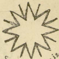
Spica Virginis.
