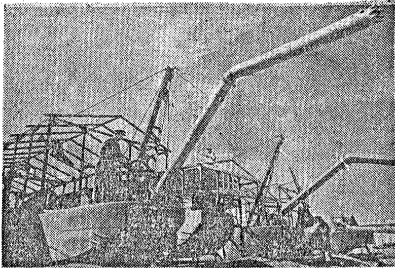
A hírközlési fűtőtorna építésénél ilyen földvájó gépek könnyítik meg a munkát.
