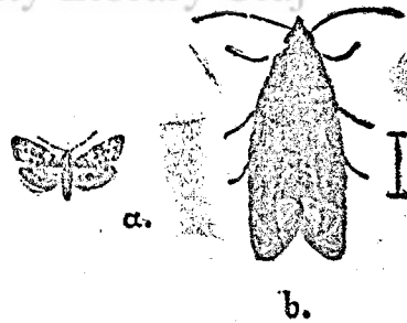
Keresztes szőlőmoly.
