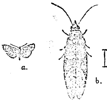
Nyerges szőlőmoly.
