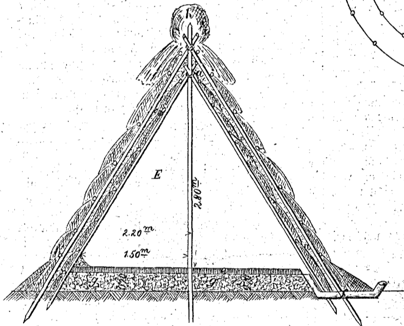
1. ábra. Jég-kunyhó. Metszet.
