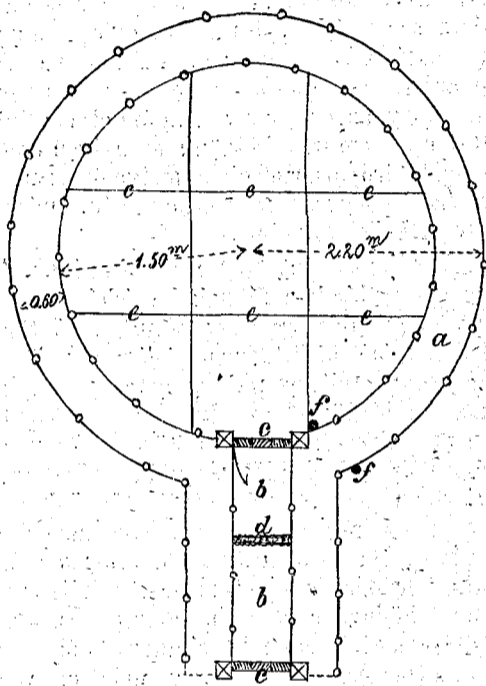
3. ábra. Jég-kunyhó. Alaprajza.
