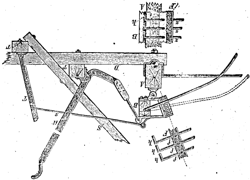
A fogakat leszorító rugó szerkezet.
