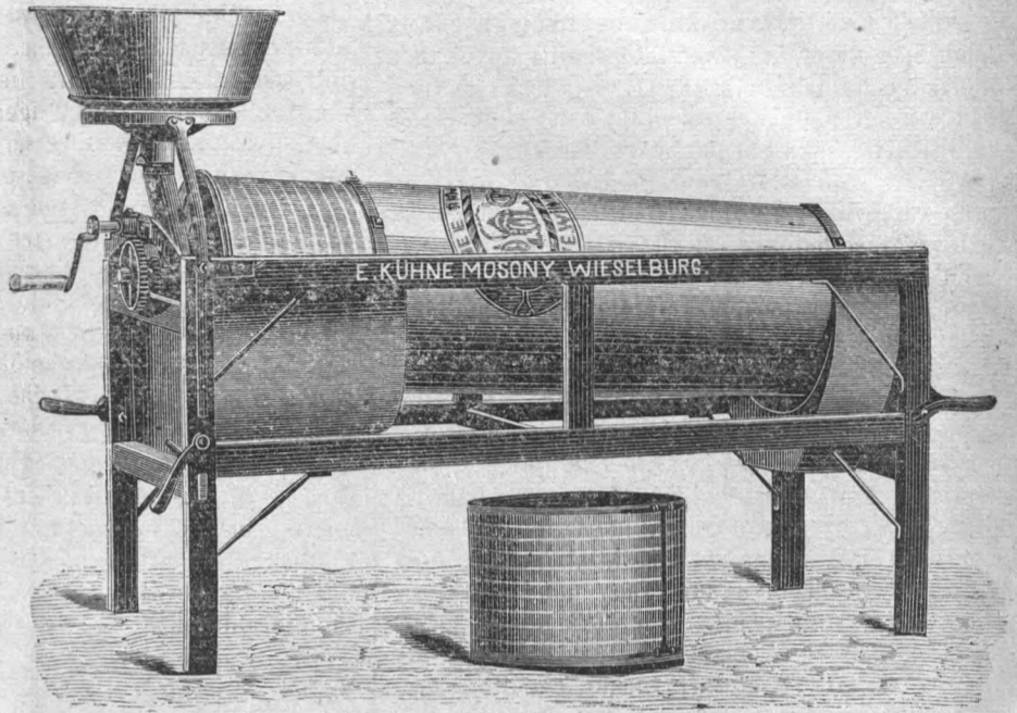
4. ábra. Pernolett-féle konkoly választógép egyszerű működéssel. Munkaképessége 5-6 hktl. óránként. Ára Bpsten 95 frt.
