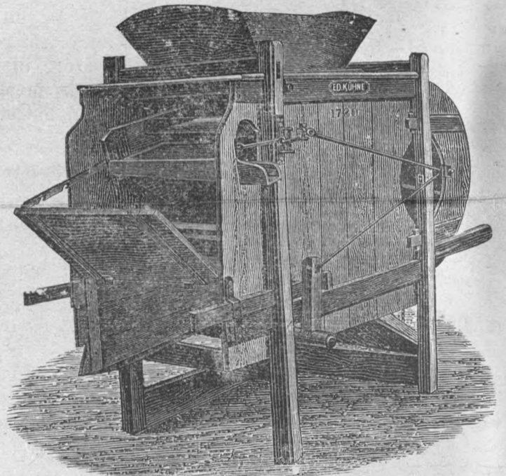
1.—2. ábra. Kühne Backer rendszerű rostái. Munkaképességük nagyság szerint 120—190 hektoliter naponta. Árak Budapesten 50—103 frt.
