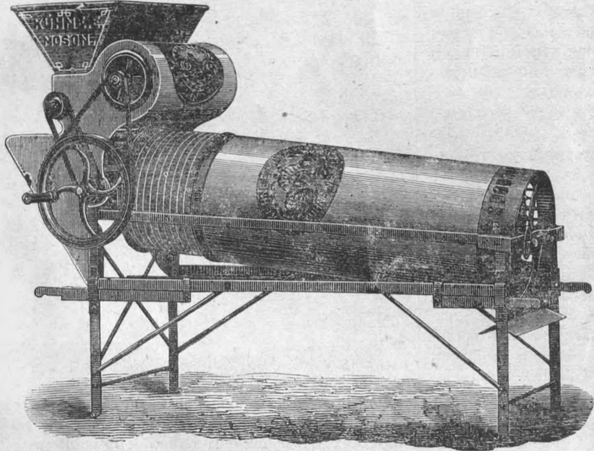
3. ábra. Vasállványos konkoly választógép szelelővel. Munkaképessége óránként 5-6 hktl. Ára Budapesten 153 frt.
